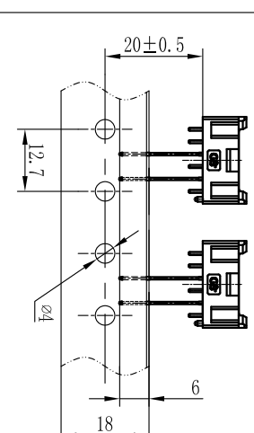
图 10-1-1 带参示意图
