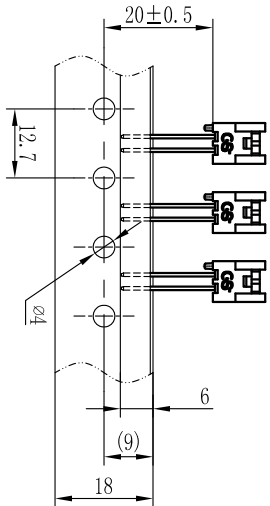
编带参考示意图
