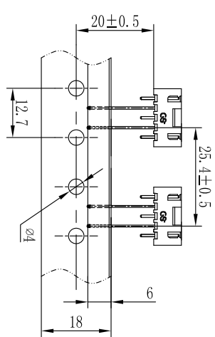
5极数编带参考示意图
