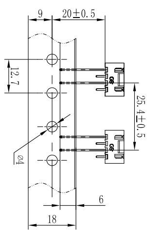
4极数编带参考示意图
